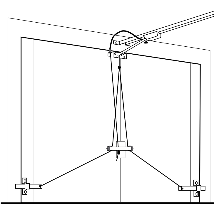
3-punktslåsning och nödfrikoppling ingår i leveransen. Låsningen är mycket genomtänkt och minskar väsentligt inbrottsrisken. Dels sker låsning i karmen i båda sidorna och dels med motorn – tre punkter således
